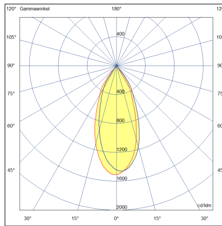
Lichtverteilungskurve SCOPE R159 40°
