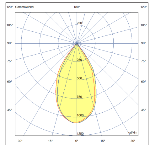
Lichtverteilungskurve SCOPE R159 55°
