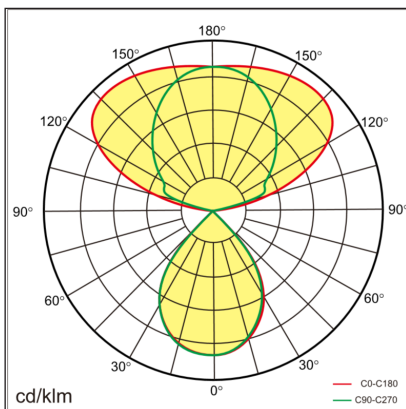
Lichtverteilungskurve SECRET SL-Q 75° direkt 150° indirekt
